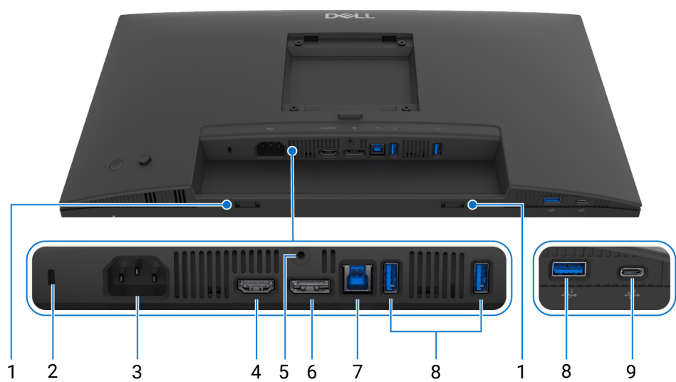
Figura 3. Vista inferior sin soporte de monitor
