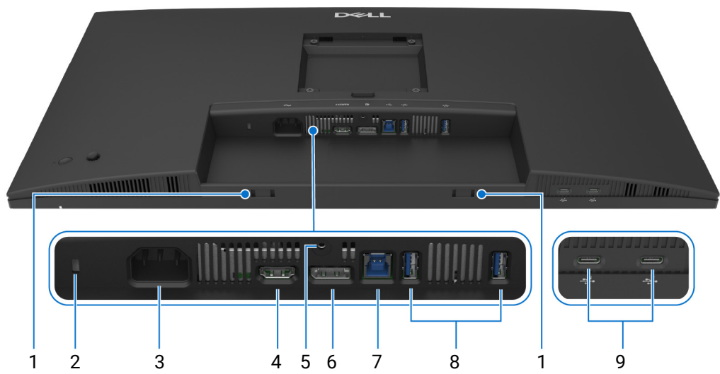
Figura 6. Vista inferior sin soporte de monitor
