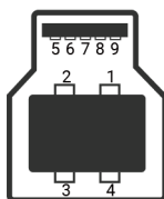
Figura 9. Conector USB Type-B
