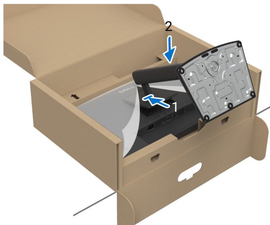
Figura 20. Fijación del soporte al monitor
