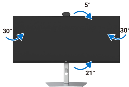
Figura 26. Ajuste de inclinación y giro (P3426WEV).
