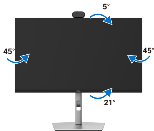
Figura 25. Ajuste de inclinación y giro (P2426HEV/P2726DEV).
