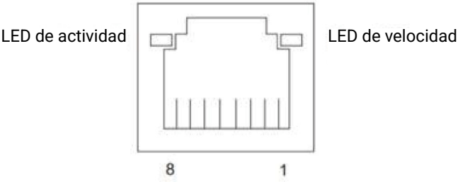
Figura 13. Puerto RJ45 (lado del conector)
