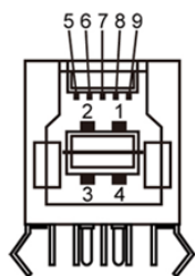
Figura 10. Puerto USB tipo B ascendente de 5 Gbps
