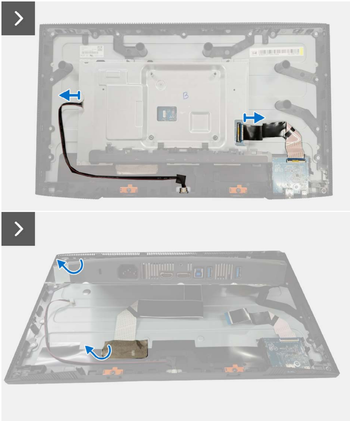
Figura 9. Retirar el protector metálico
