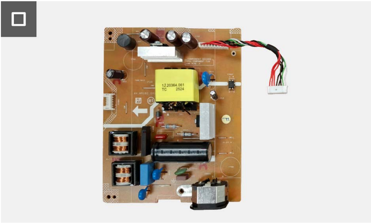
Figura 18. Retirar la placa de alimentación
