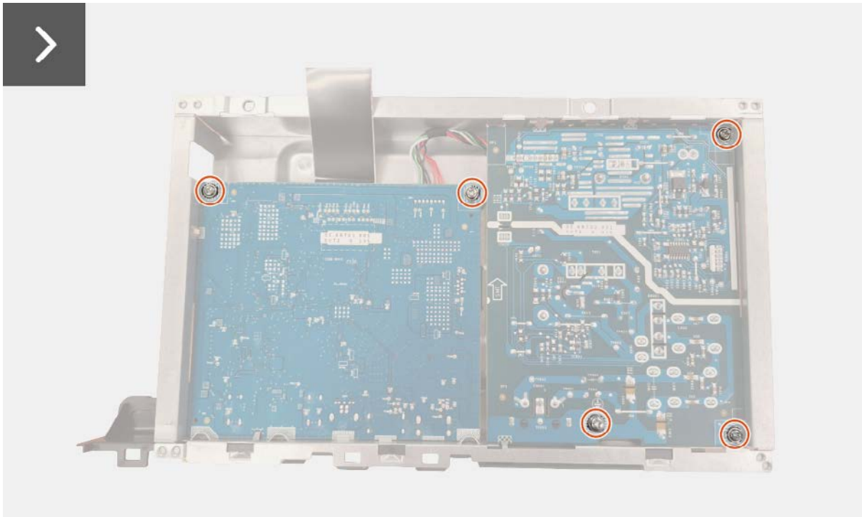
Figura 20. Instalar la placa de alimentación
