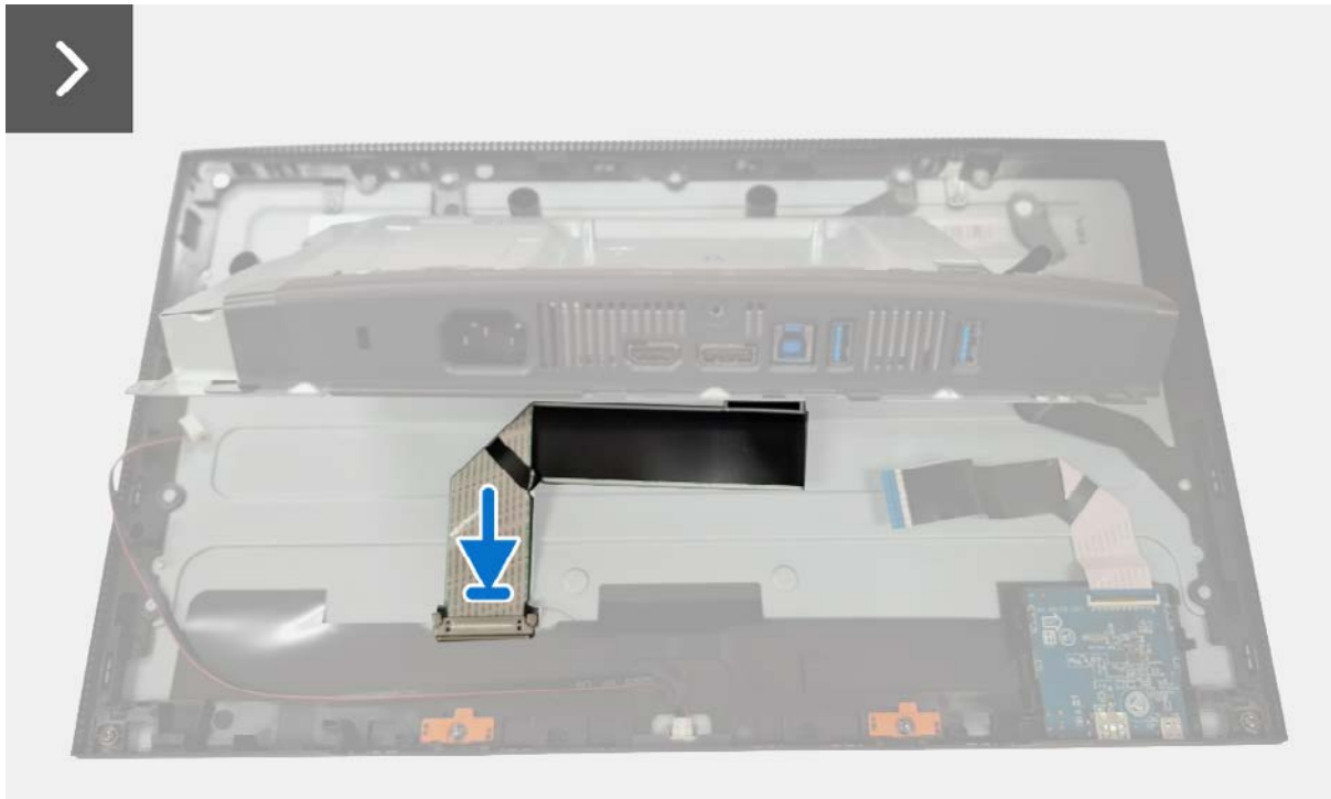
Figura 12. Instalar el protector metálico
