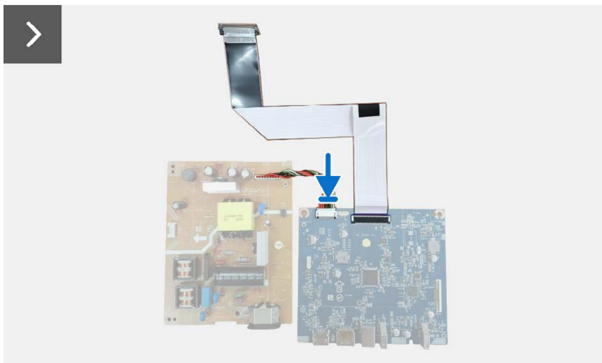
Figura 19. Instalar la placa de alimentación
